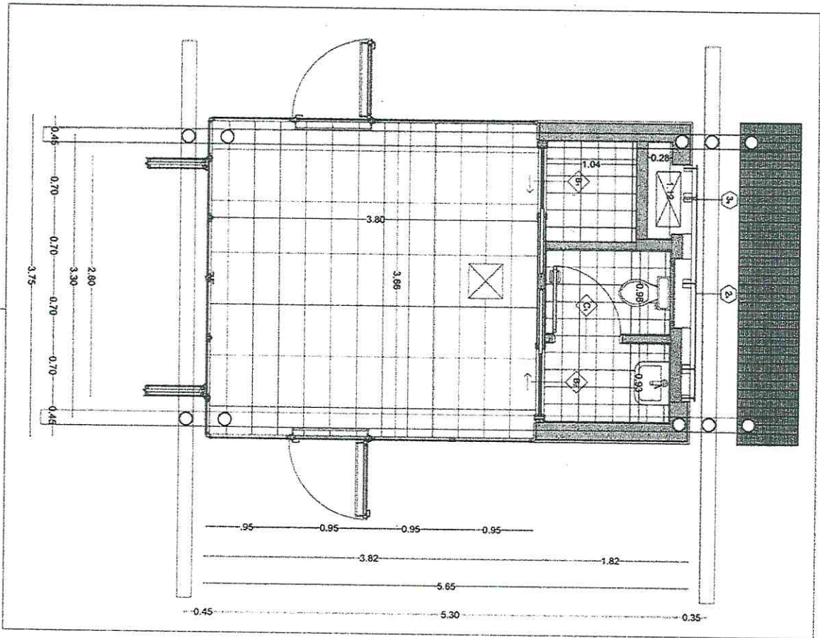
Pianta Gazebo A.D
